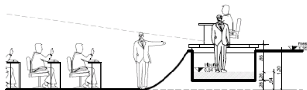
CORTE TRIBUNA
