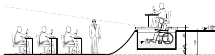
CORTE TRIBUNA
