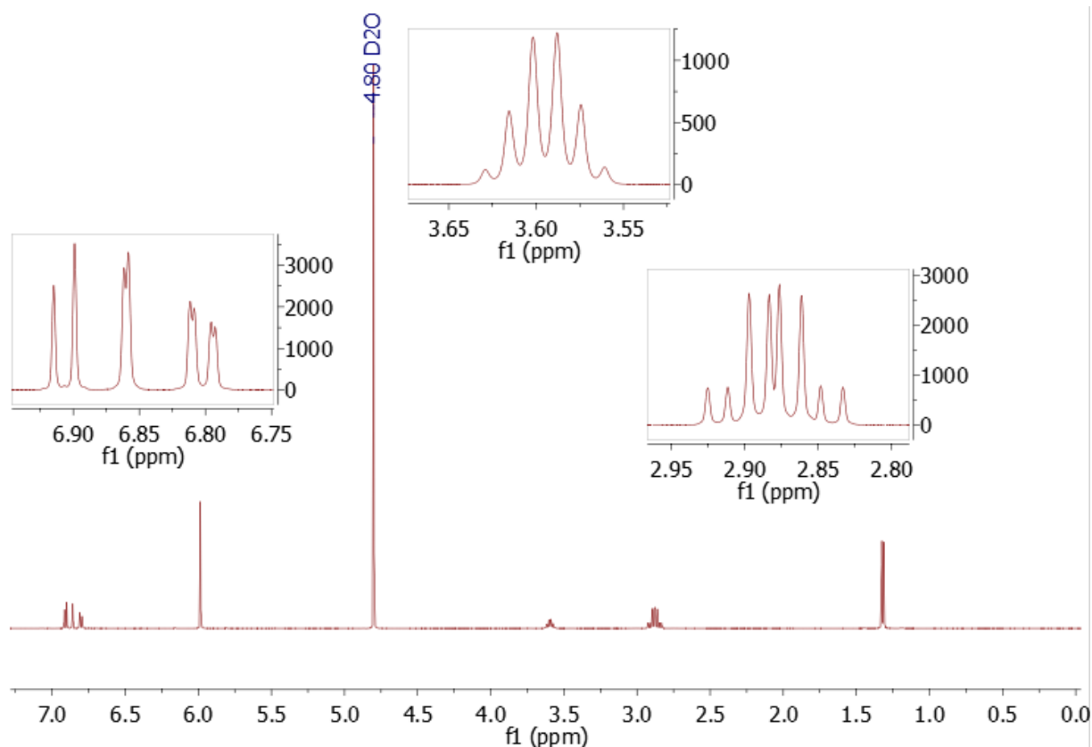
Figura 1: Espectro de RMN de 1 H a 500 MHz para o MDA.HCl em D 2 O
