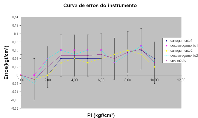
FIGURA 2– Curva de erros do instrumento calibrado
