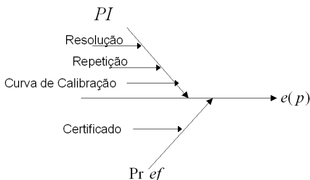
FIGURA 3 - Diagrama causa - efeito da calibração de um Transdutor/Transmissor de pressão
