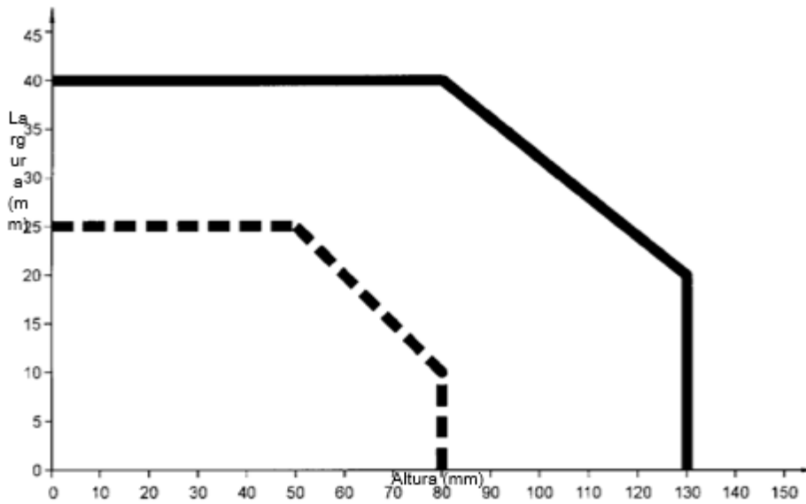
Gráfico da Tabela 2 (pneu radial) AVARIA NA ÁREA DOS FLANCOS TAMANHO MÁXIMO A CONSERTAR
