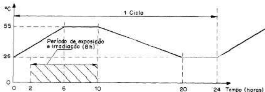
Figura 6 - Ciclo de exposição à radiação solar
