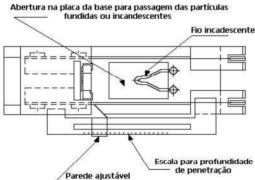
Figura 9 - Aparelho para ensaio de exposição ao calor e ao fogo
