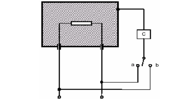
图 2 单相电动机在工作温度下泄漏电流的测量电路图
