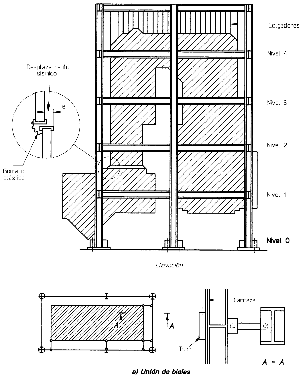
Figura A.7 - Detalles típicos de grandes equipos suspendidos, conectores sísmicos y pernos de anclaje (continúa)
