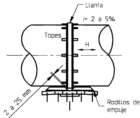
DETALLE 1 Apoyo longitudinal
